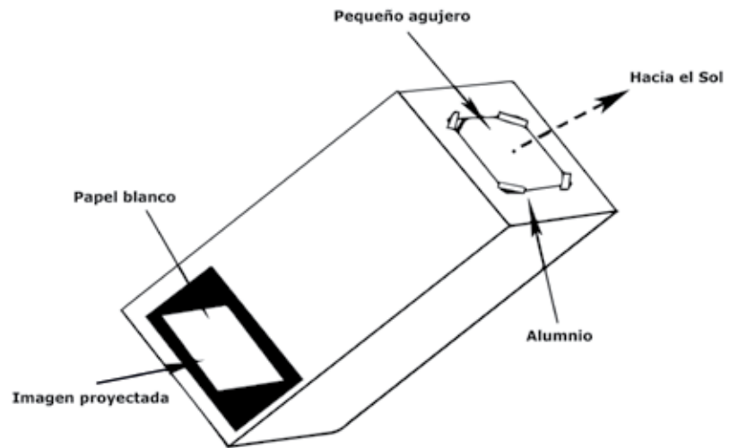
Figura 3. Proyector de eclipses
